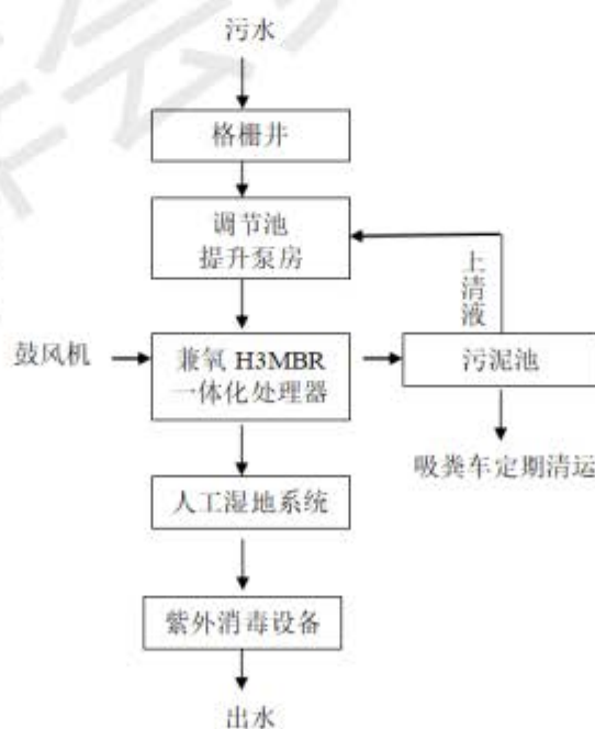
图 8 污水处理工艺流程
