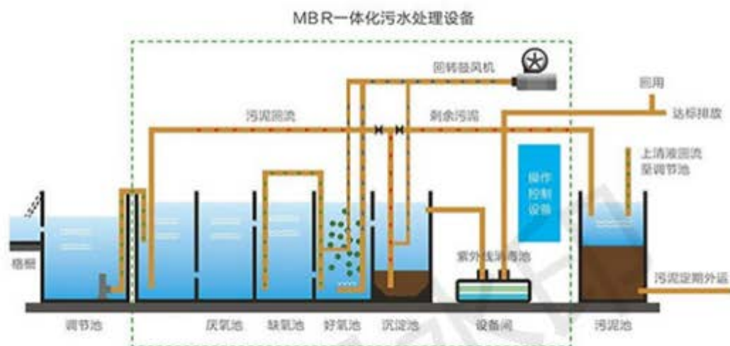
图 7 兼氧 H3MBR 工艺示意图
