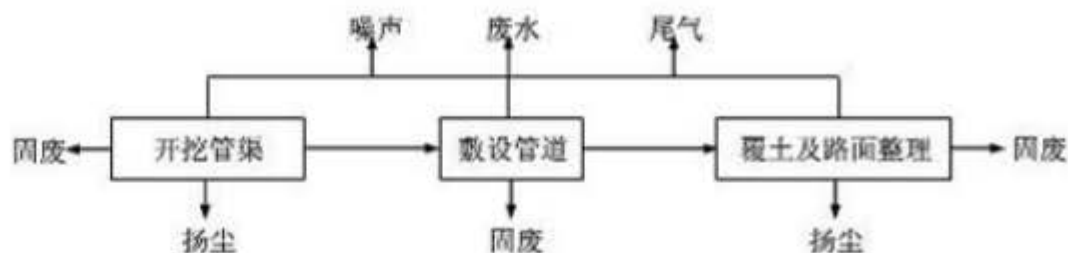
图6 配套管网工艺流程
