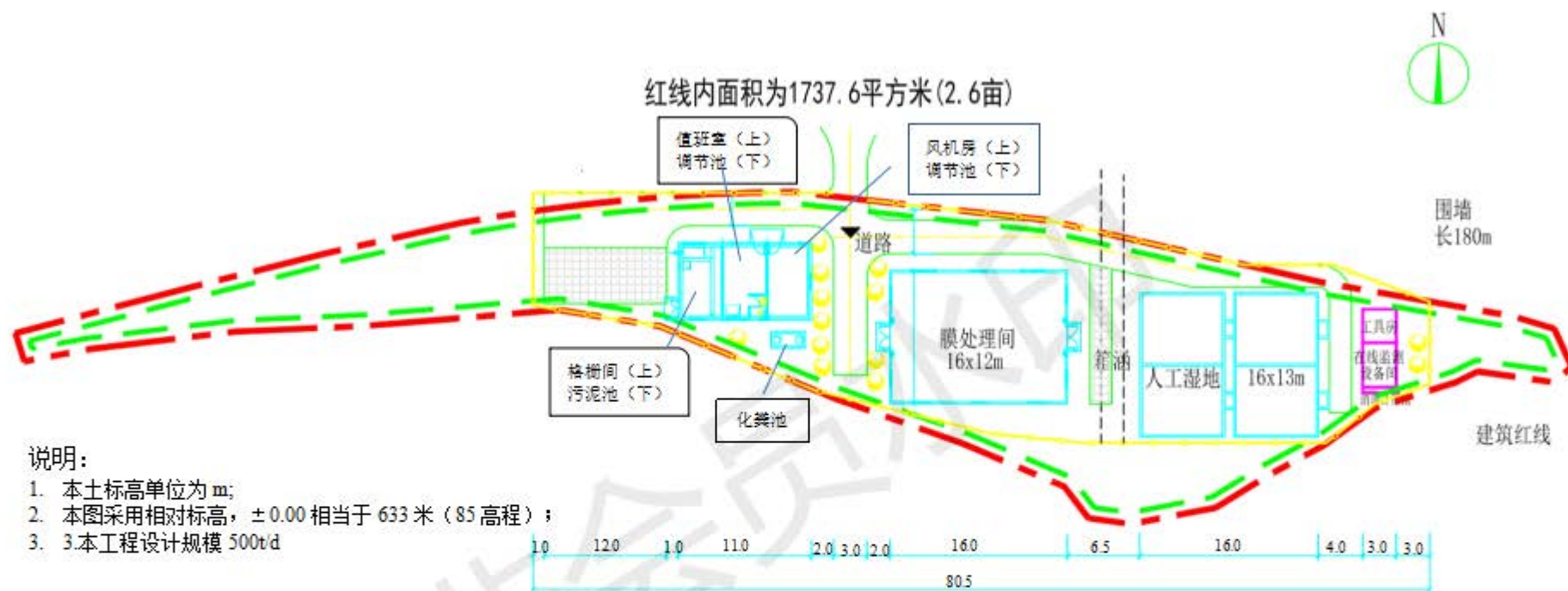
图3 洛阳镇污水处理厂平面布置图
