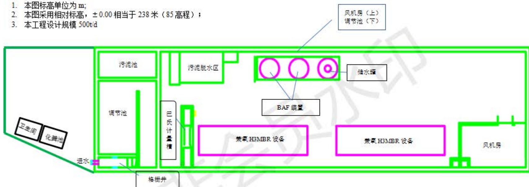
图 3 必背镇污水处理厂平面布置图
