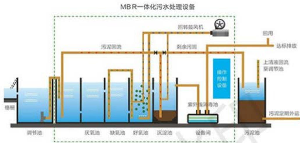
图 7 兼氧 H3MBR 工艺示意图
