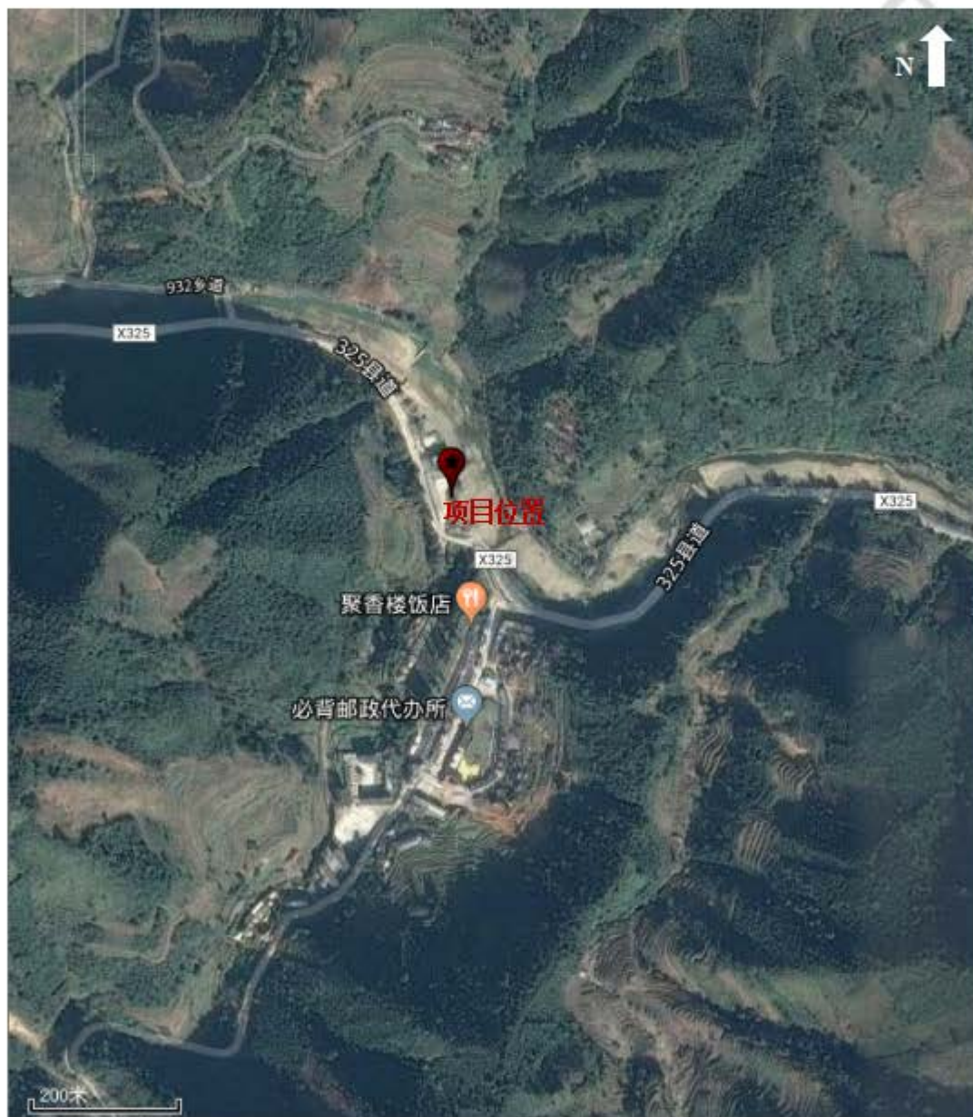
图1 必背镇污水处理厂地理位置示意图
