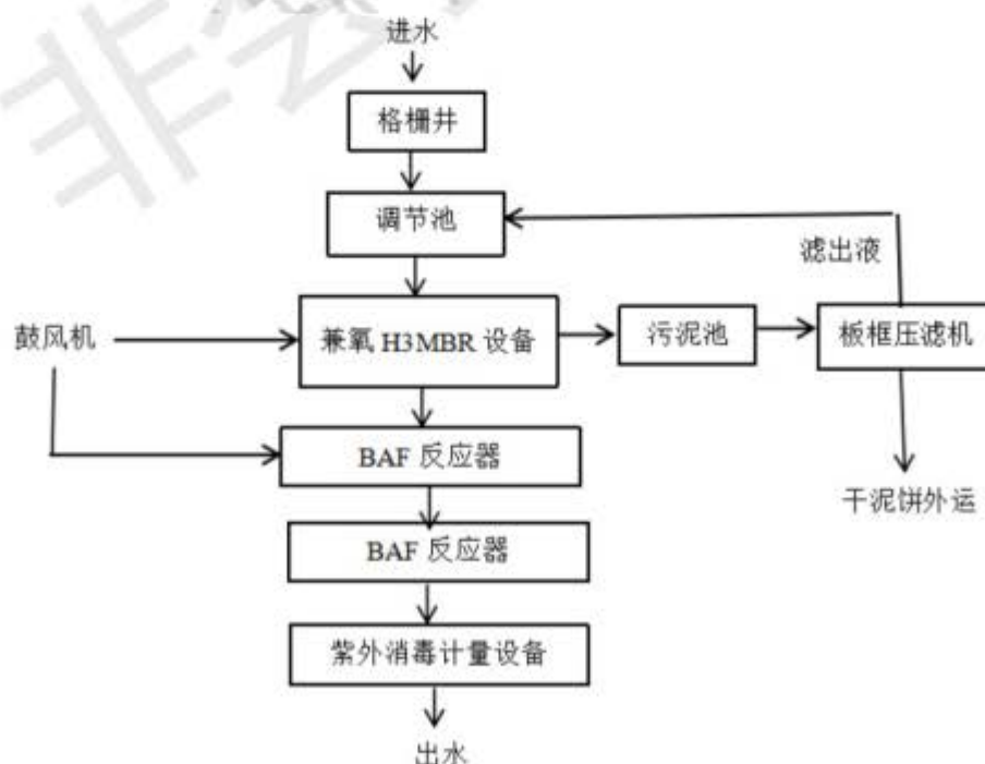
图 8 污水处理工艺流程
