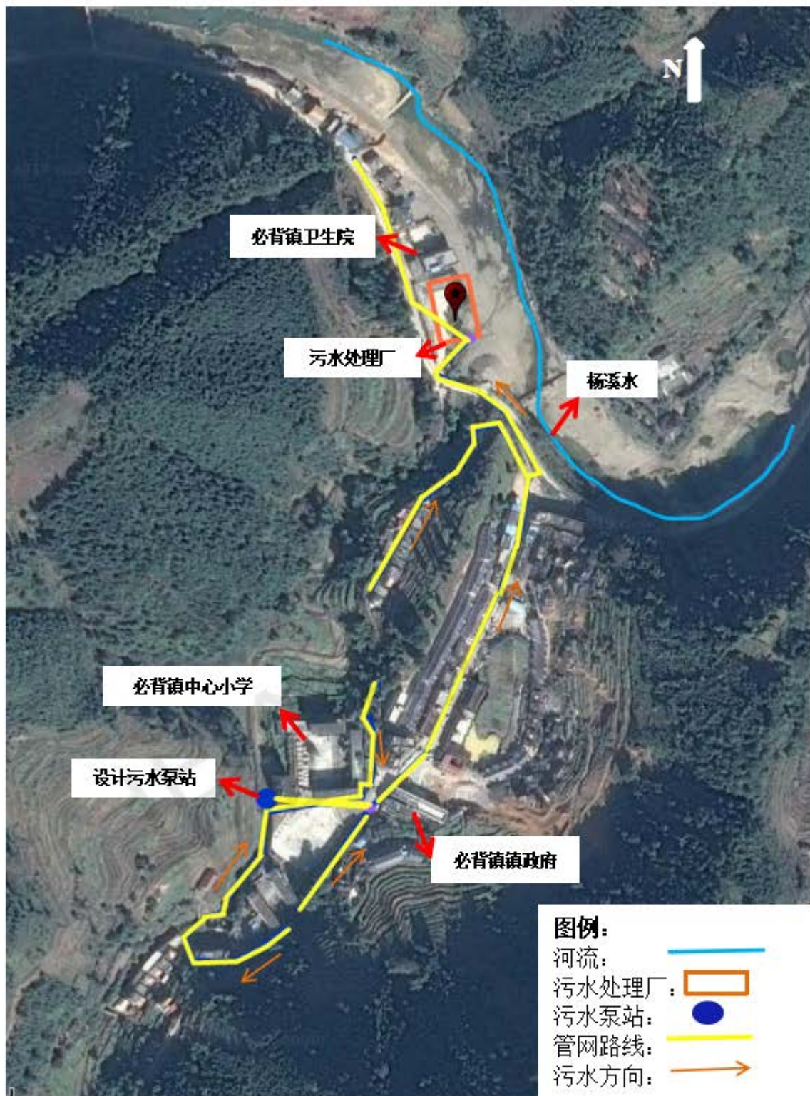
图 4 必背镇污水处理厂配套管网路线图
