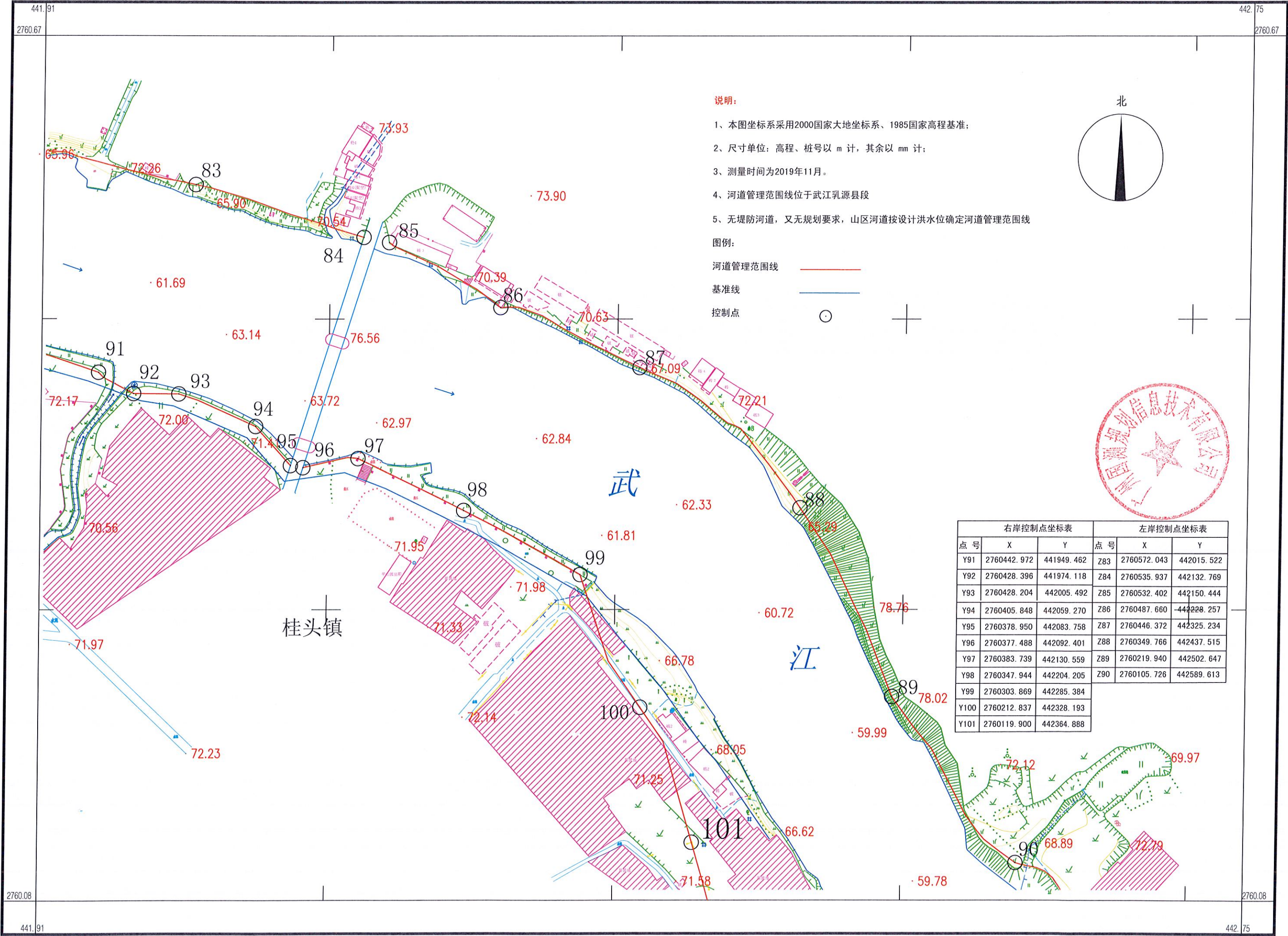
武江河乳源县河段河道管理范围划分图（26/21）
