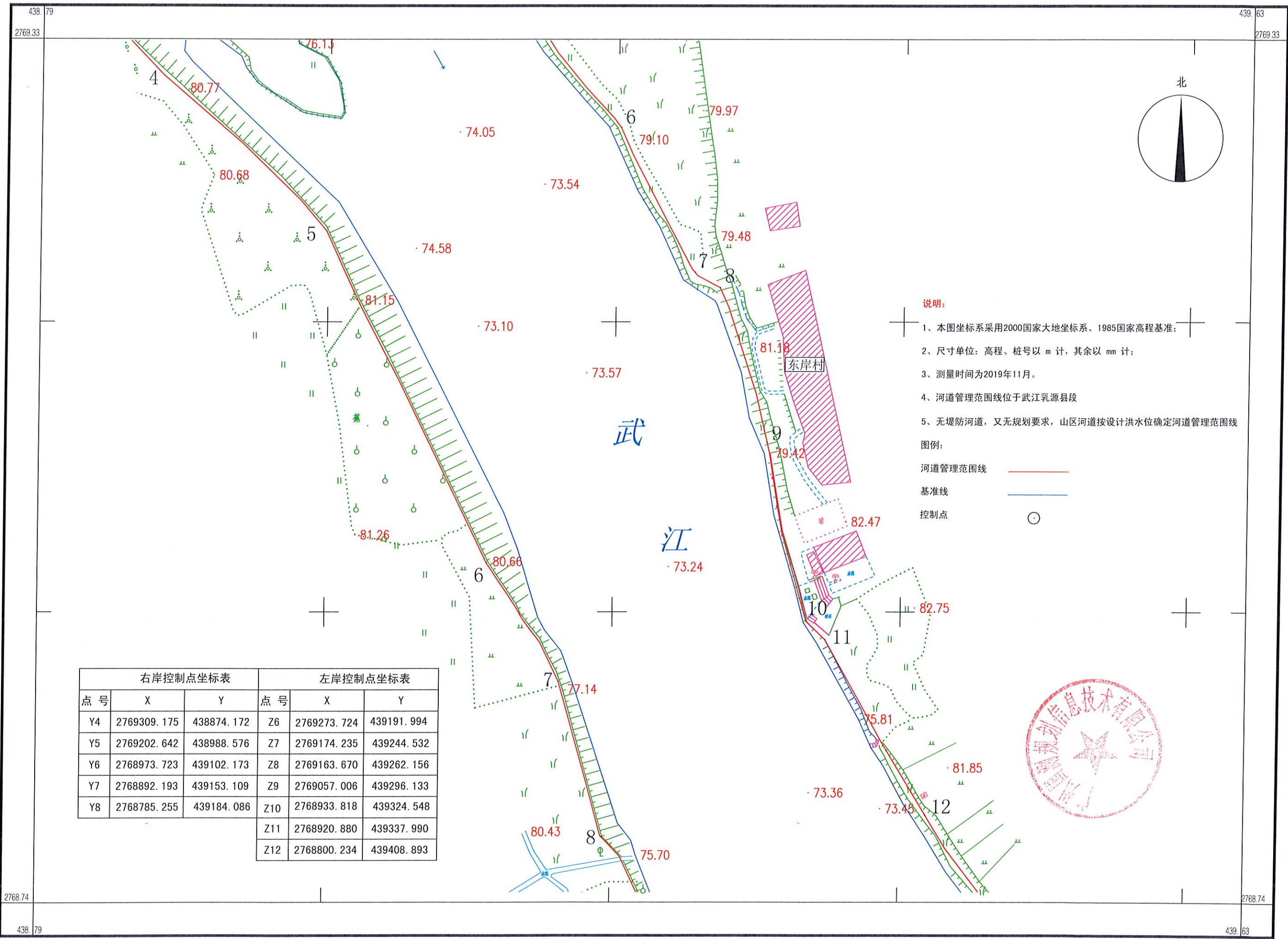
武江河乳源县河段河道管理范围划分图（26/2）
