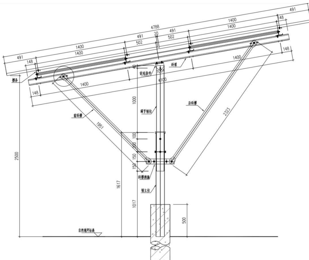
图 3 光伏支架示意图
