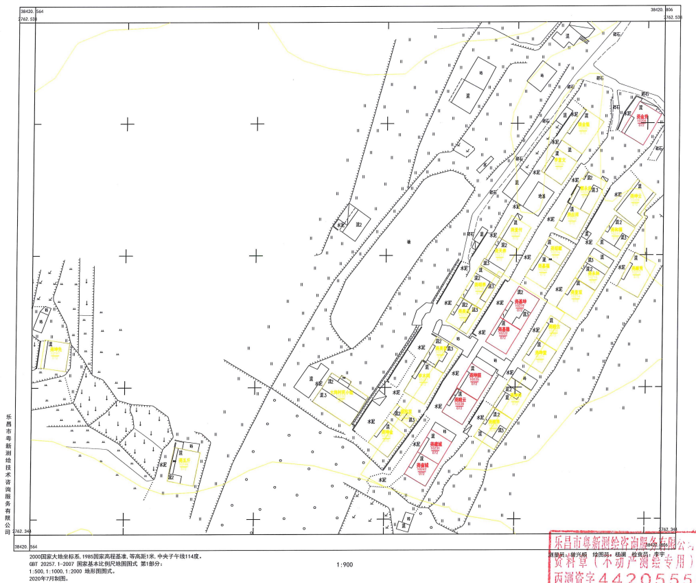
乳源县大桥镇大桥村委会长山子村“房地一体”公示图一 2762.34-38420.56
