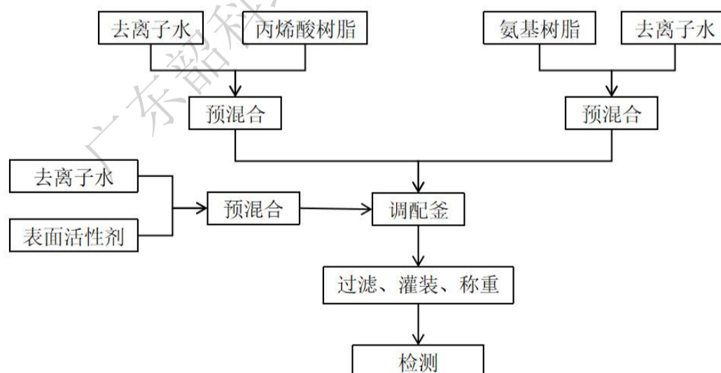
图 2-4 02 号水性涂料生产线工艺流程图
