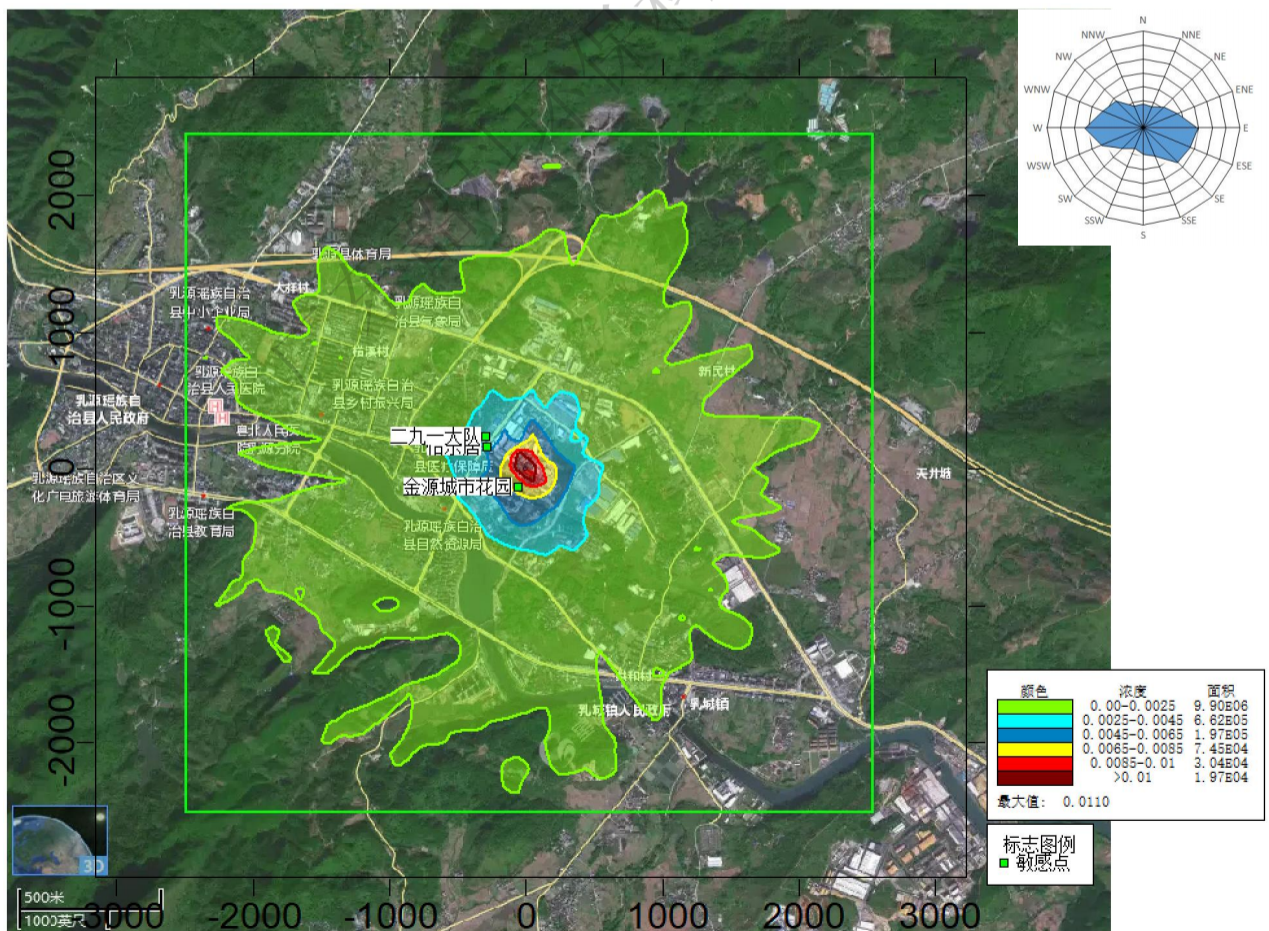
图 4-7 正常排放非甲烷总烃小时平均浓度各点贡献值分布图 ( \text{mg}/\text{m}^3 )
