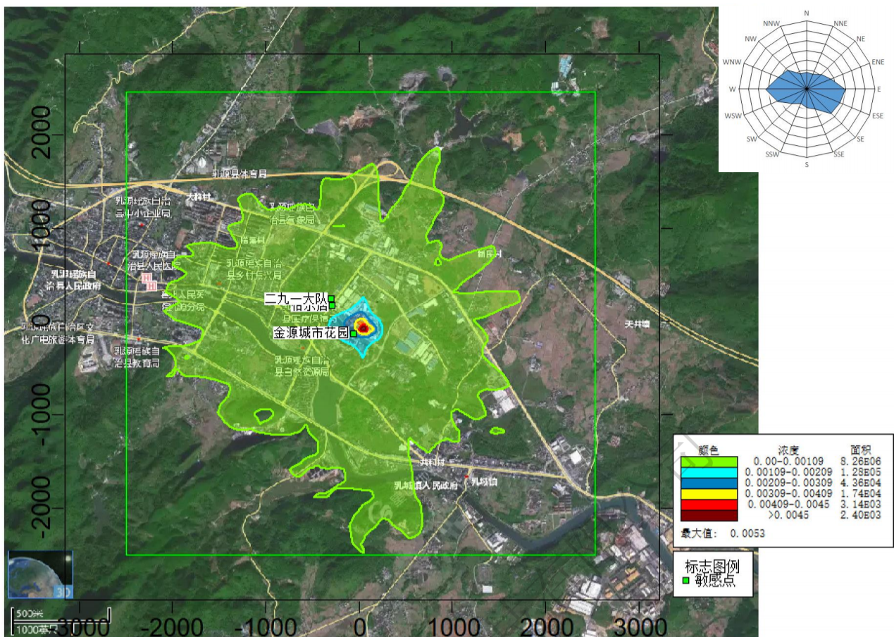
图 4-6 正常排放 TVOC 小时平均浓度各点贡献值分布图 ( \text{mg}/\text{m}^3 )
