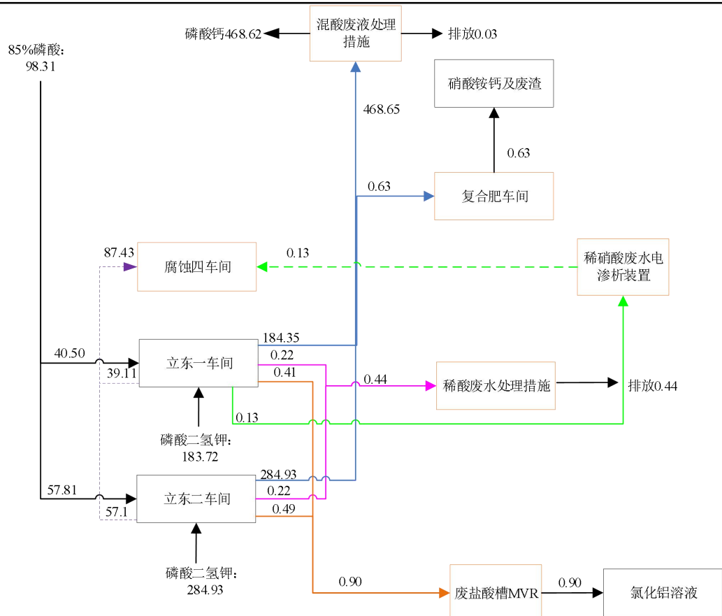
图 5 现有工程（已建+拟建技改工程）全厂磷元素平衡图（t/a）
