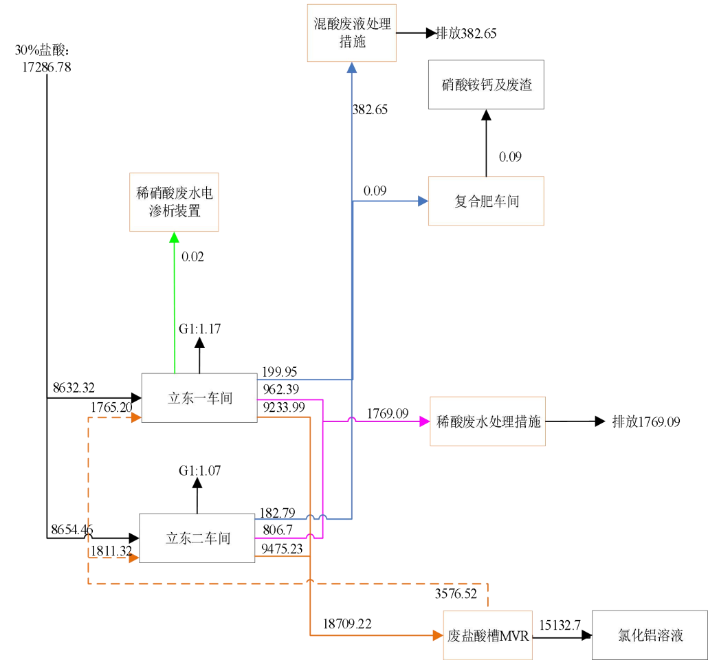
图 4 现有工程（已建+拟建技改工程）全厂氯元素平衡图（t/a）
