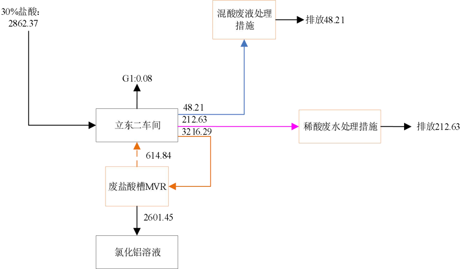
图 13a 扩建工程氯元素平衡图（t/a）
