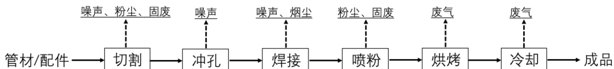
图6 生产工艺流程及产污环节图
