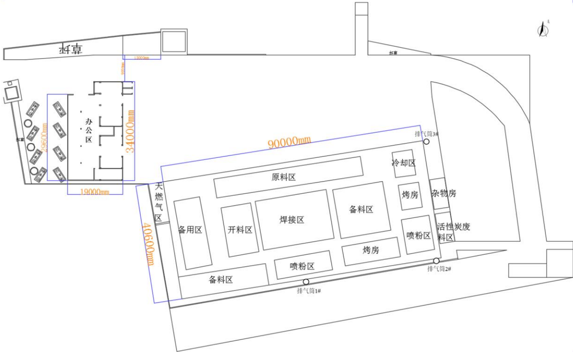
图 3 生产厂区平面布置图
